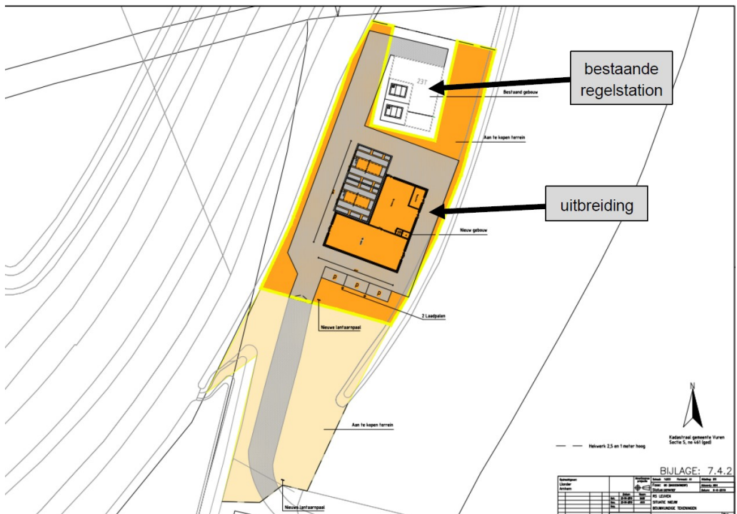
Toekomstige situatie elektriciteitsregelstation Leuven (noorden is links)
