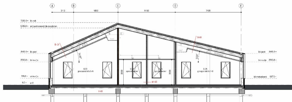
Doorsnede A
