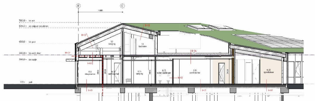
Doorsnede E
