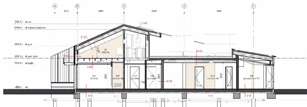
Doorsnede D
