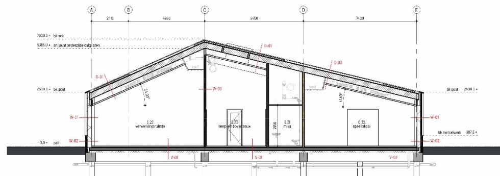
Doorsnede B
